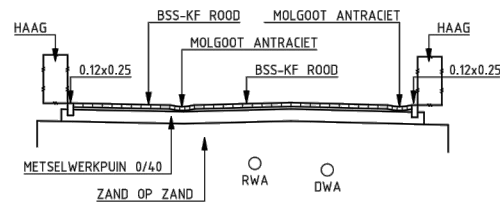
PRINCIPE PROFIEL 1 SCHAAL 1:100
